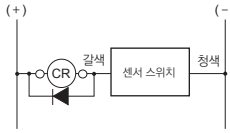
AND(직렬)연결, OR(병렬)연결
