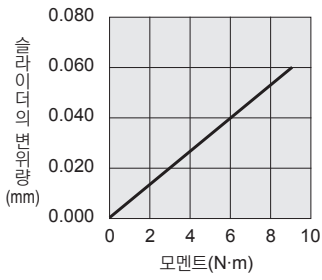
피칭 방향 모멘트(Mp)
