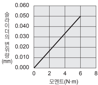
피칭 방향 모멘트( M_p )
