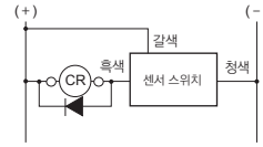
AND(직렬)연결, OR(병렬)연결
