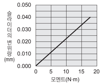
요잉 방향 모멘트(My)
