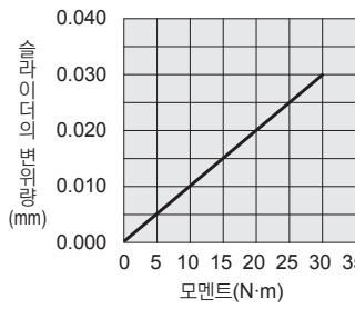
롤링 방향 모멘트(Mr)
