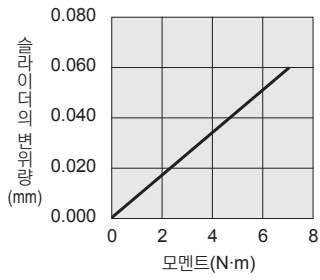
롤링 방향 모멘트(Mr)
